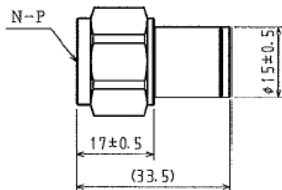
*外観図
