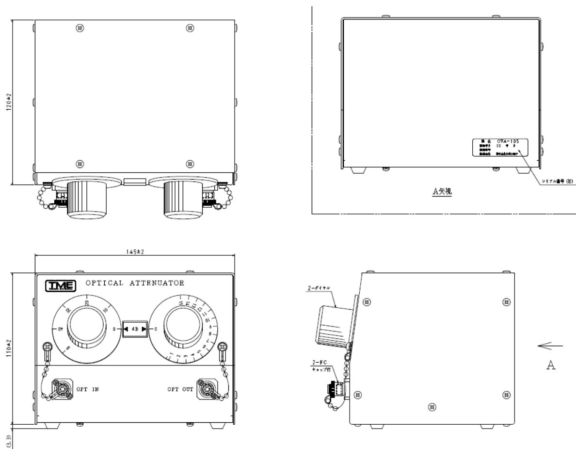
図3 製品外観
